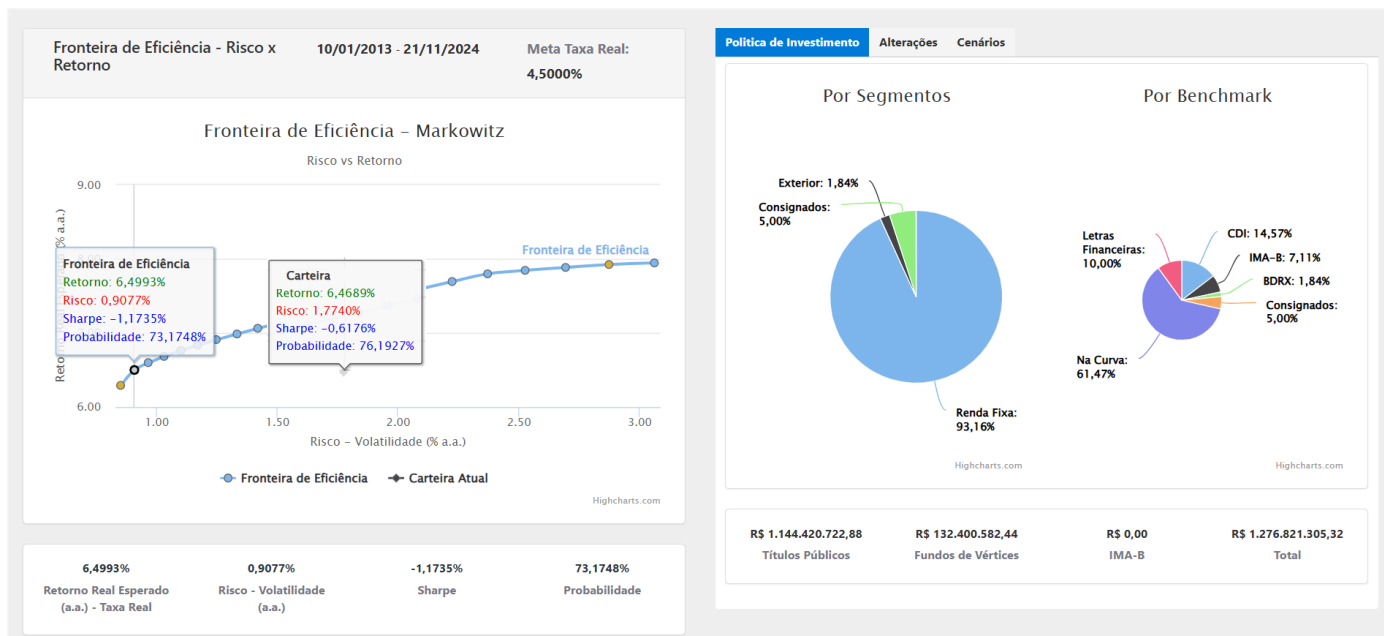
Figura 05 - Fronteira de Eficiência - Markowitz
