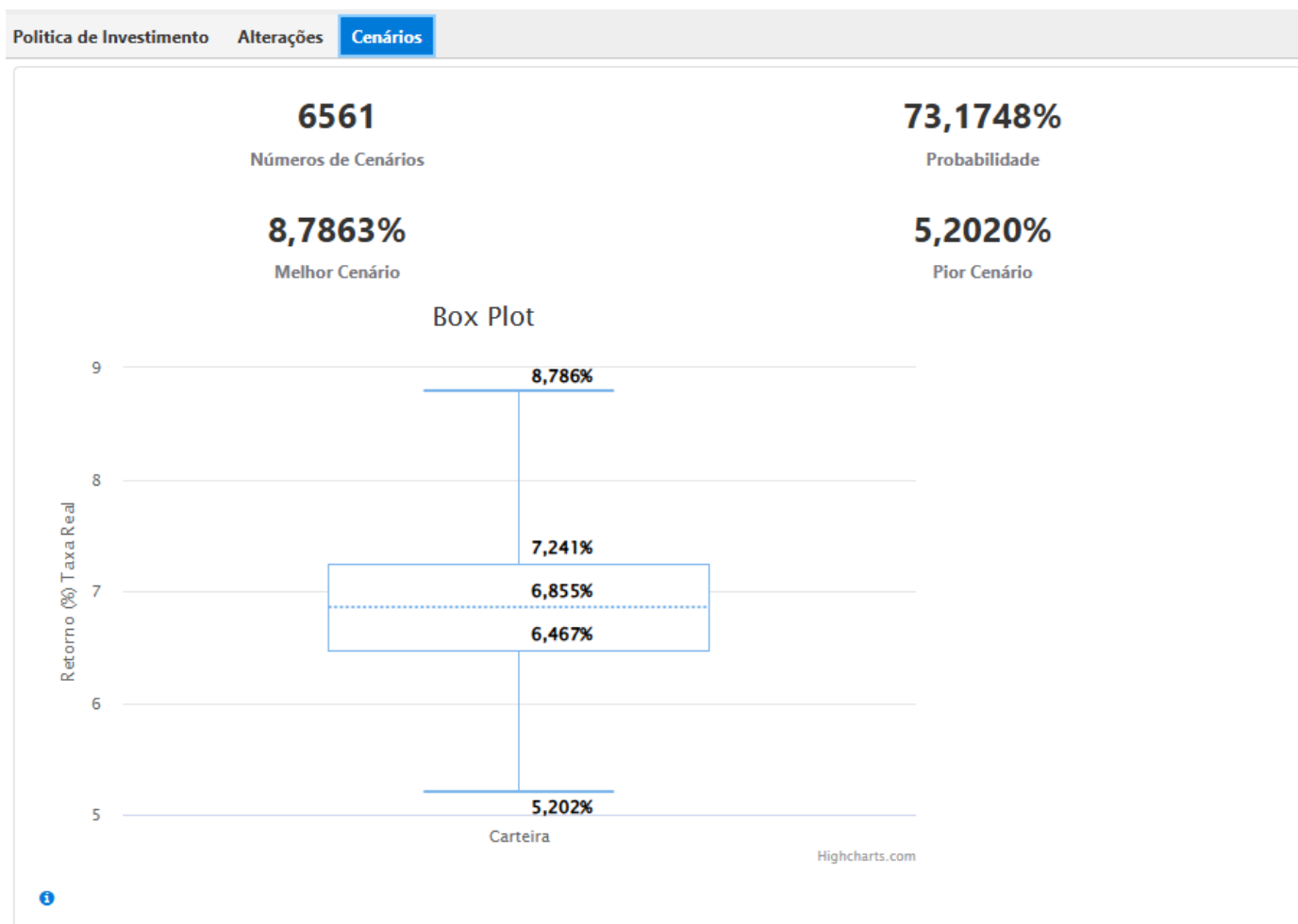
Figura 07 A - Gráfico Box Plot - Cenários
