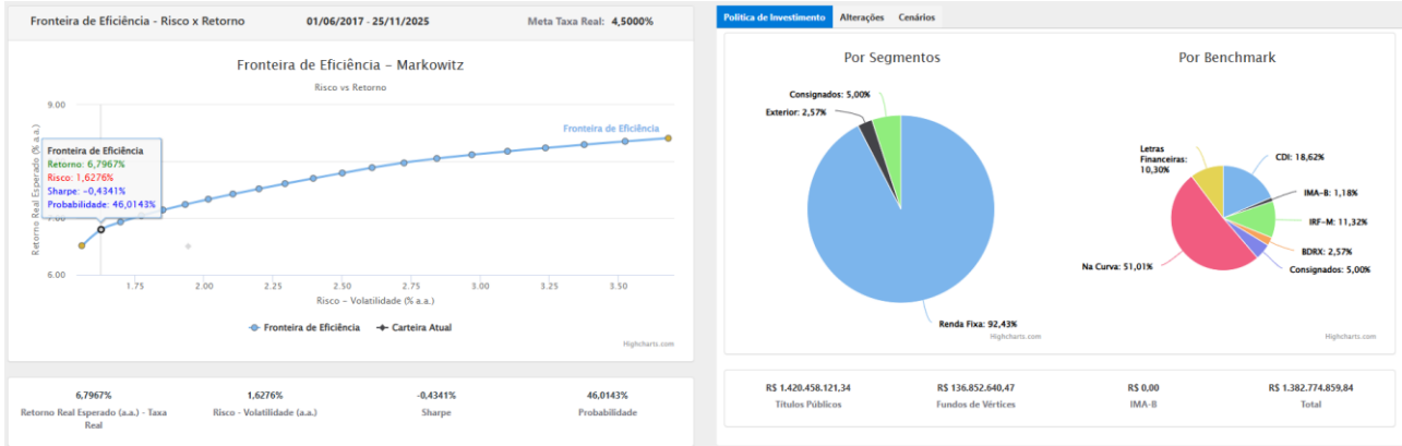
Figura 05 - Fronteira de Eficiência - Markowitz
