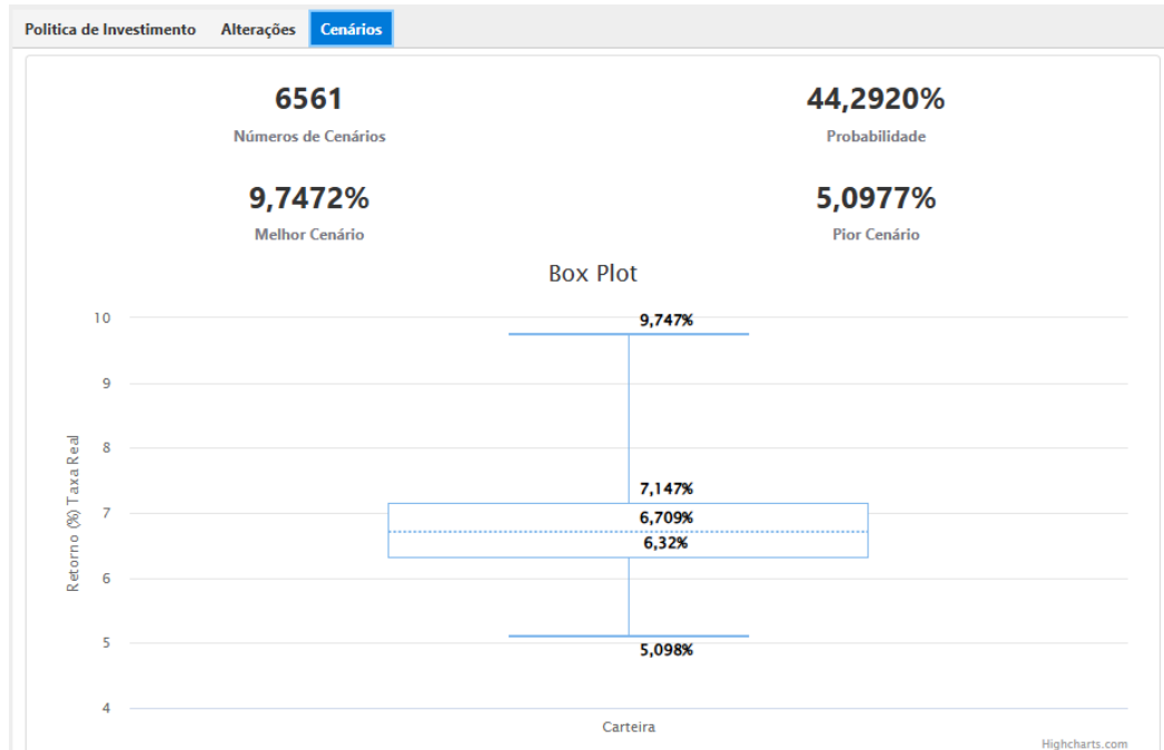
Figura 07 A - Gráfico Box Plot - Cenários
